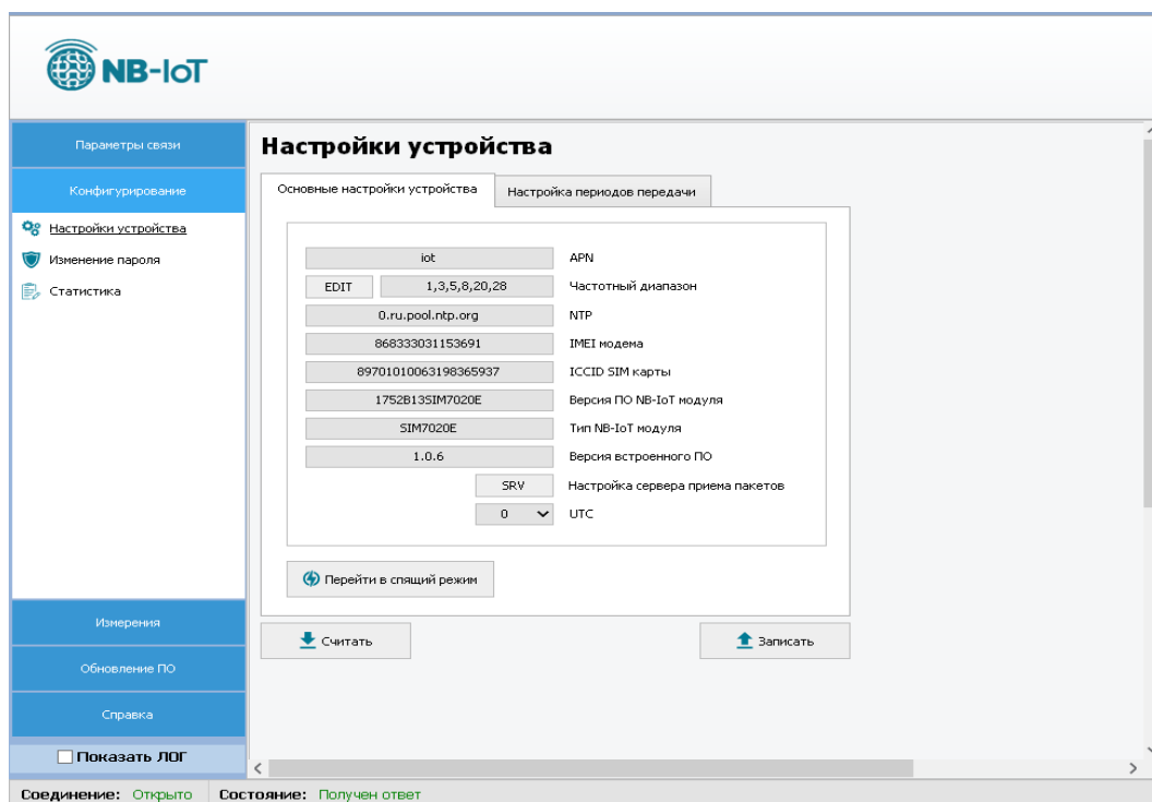
Рис. 6 – Вкладка «Настройка устройства»
